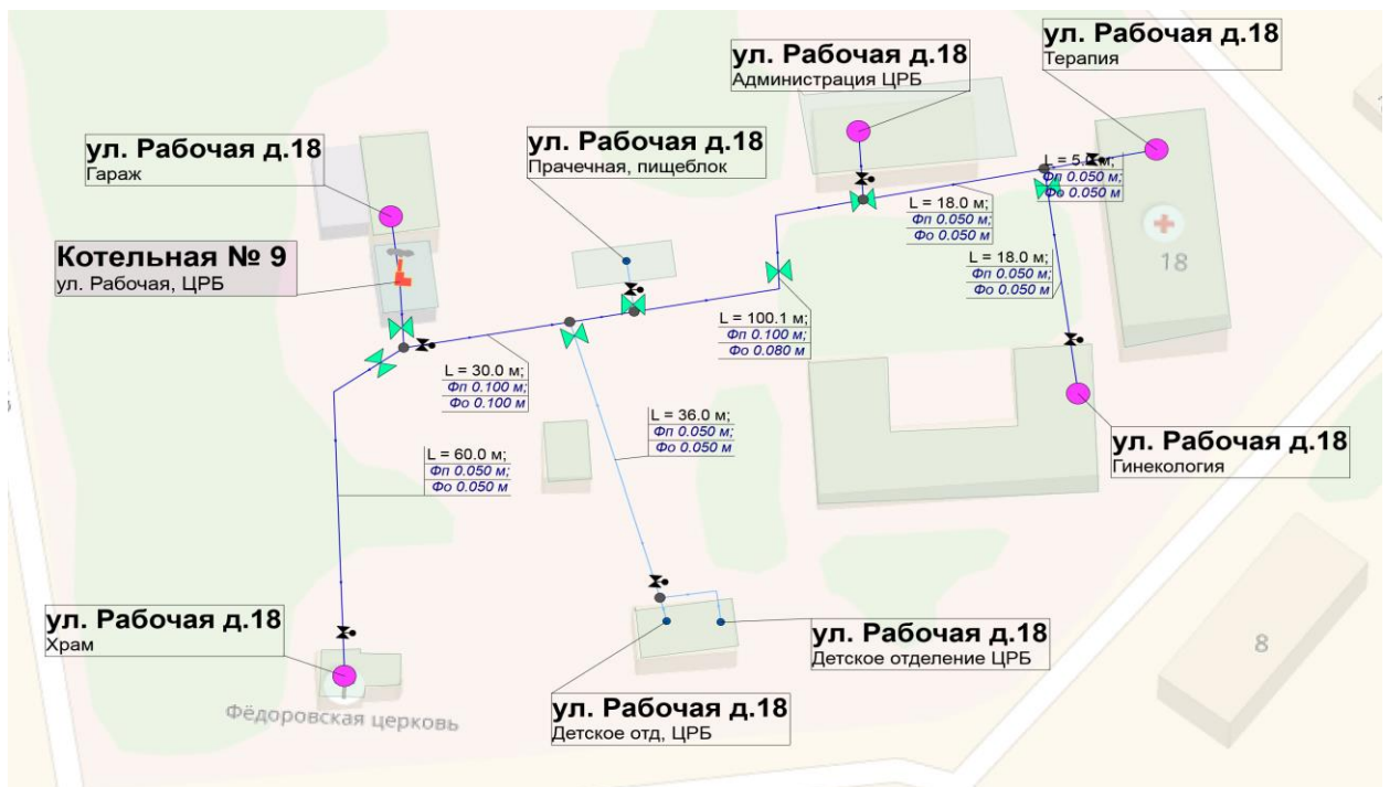
Рисунок 1.3 – Схема тепловых сетей котельной № 9 п. Парфино, ул. Рабочая ЦРБ
