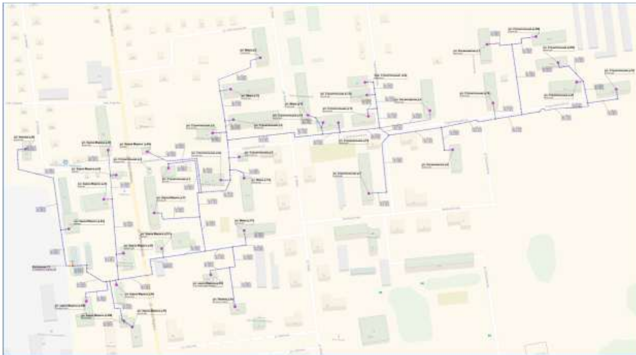
Рисунок 6. Схема тепловых сетей котельной №13
