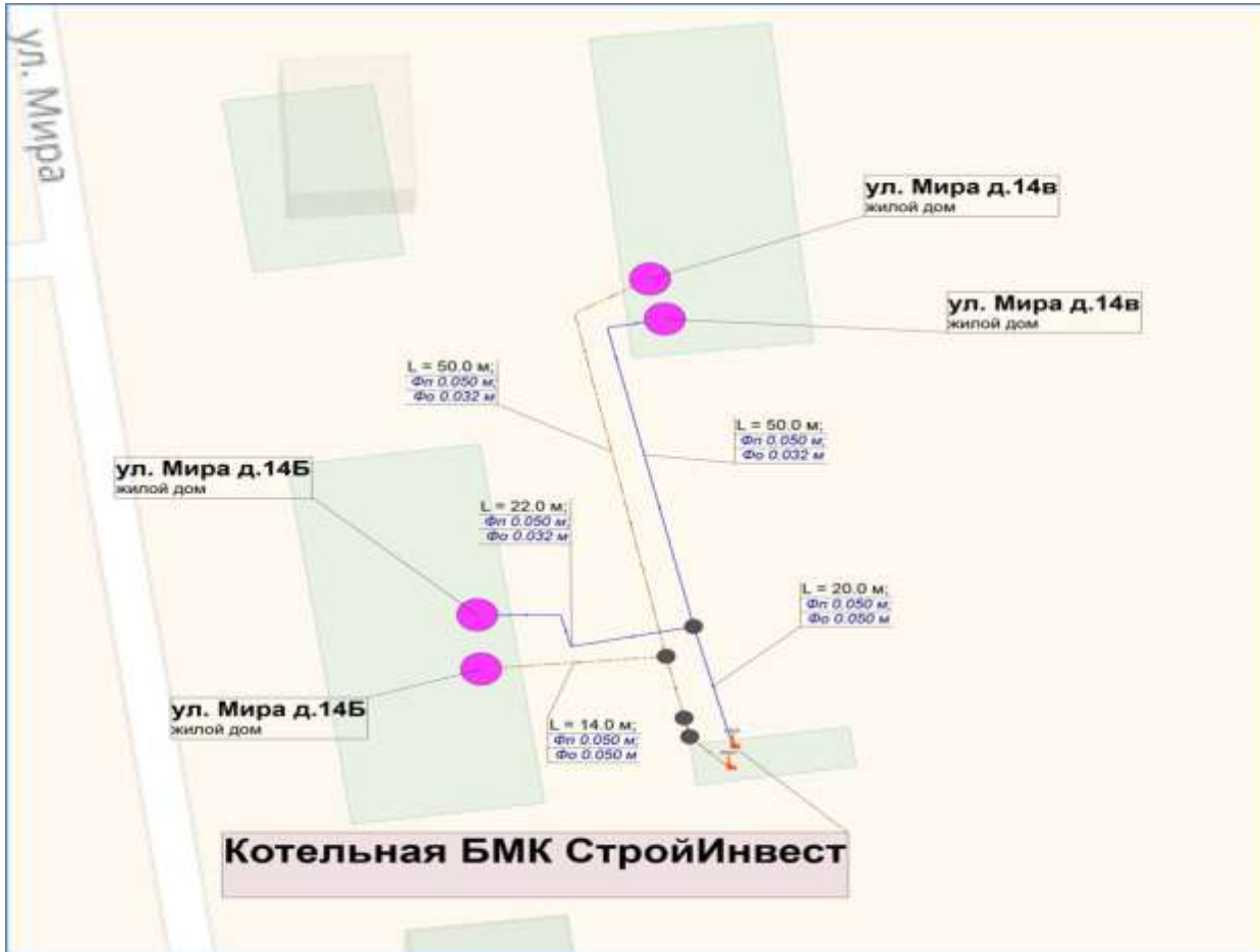
Рисунок 5. Схема тепловых сетей БМК "Стройинвест"
