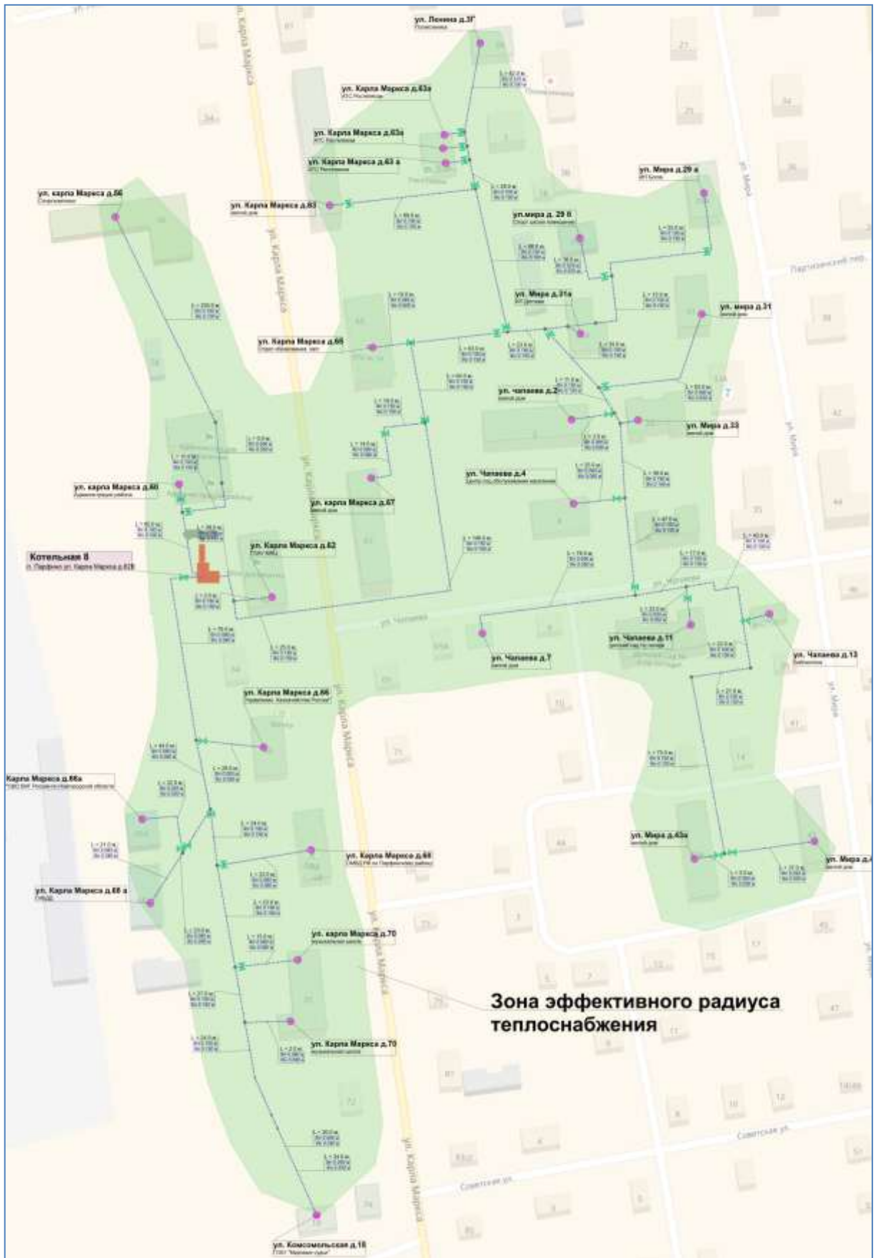
Рисунок 8: Зона эффективного радиуса теплоснабжения котельной №8
