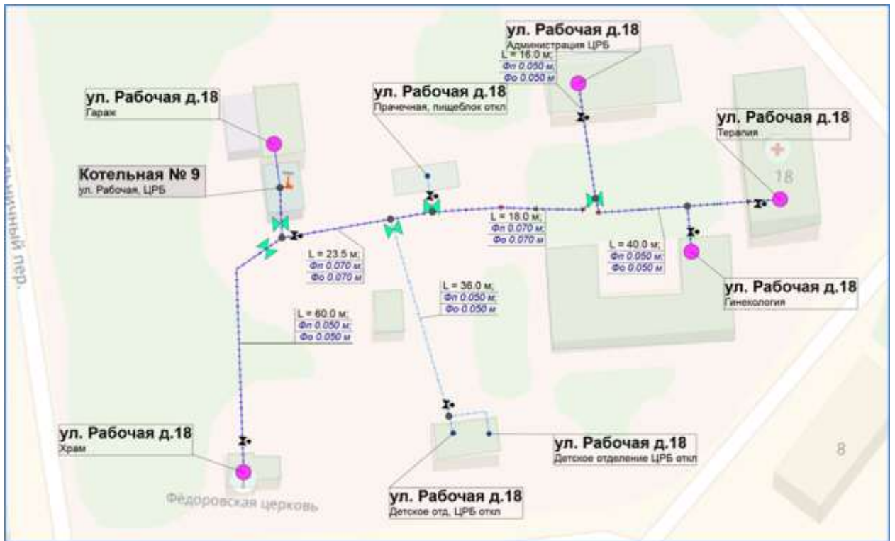
Рисунок 3. Схема тепловых сетей котельной №9
