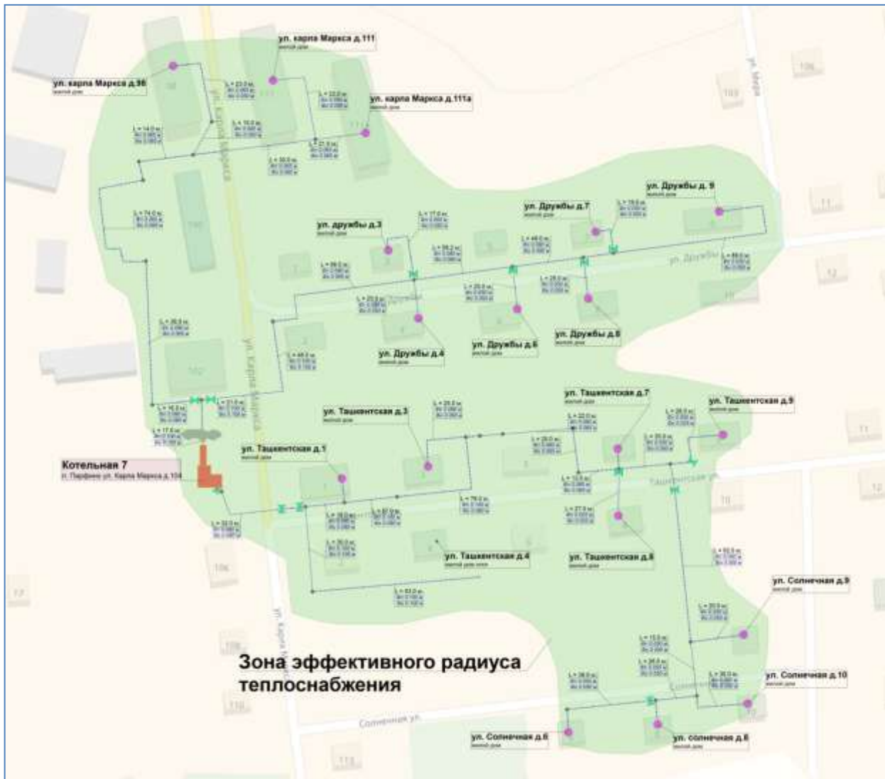
Рисунок 7: Зона эффективного радиуса теплоснабжения котельной №7
